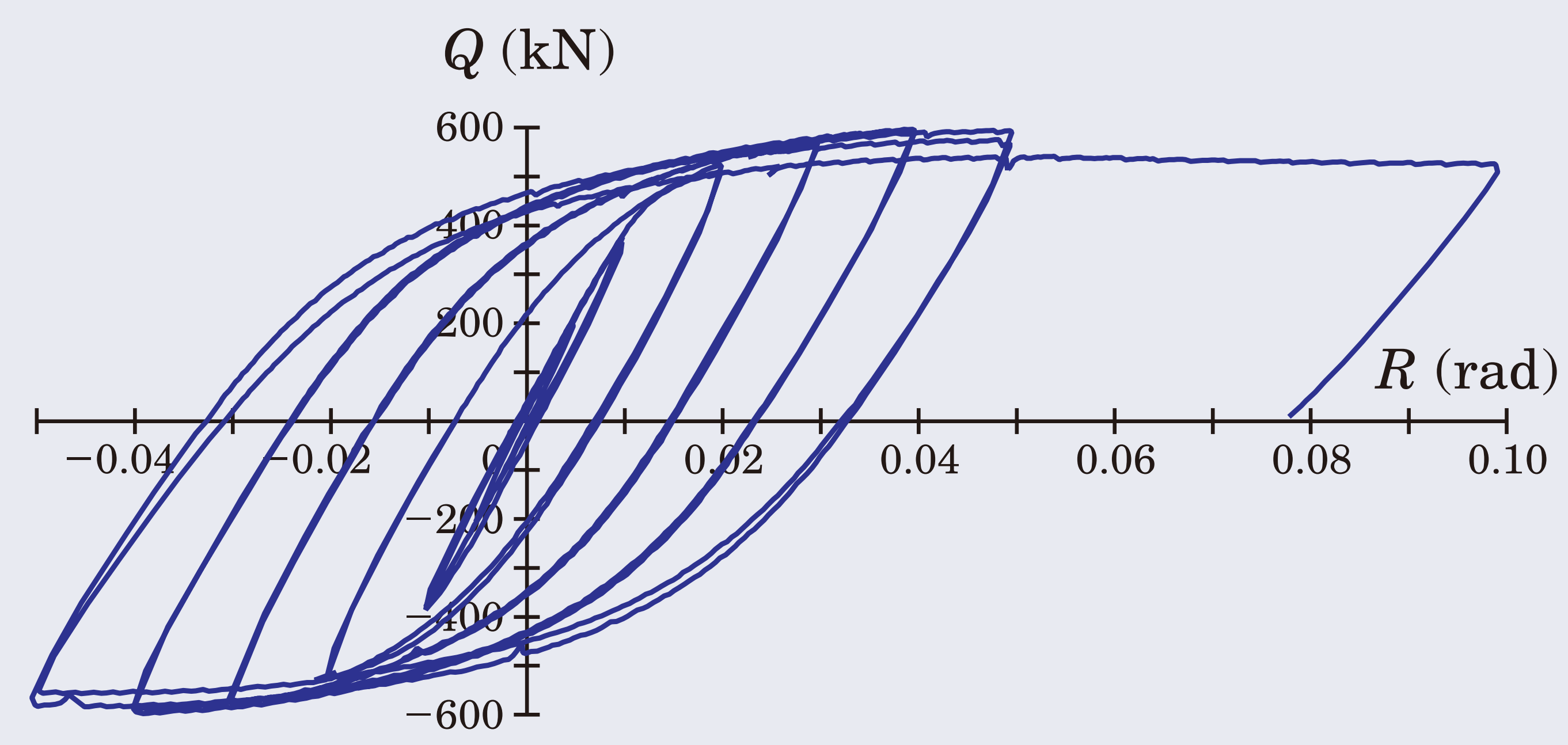
実験結果（スパン6.0m）
