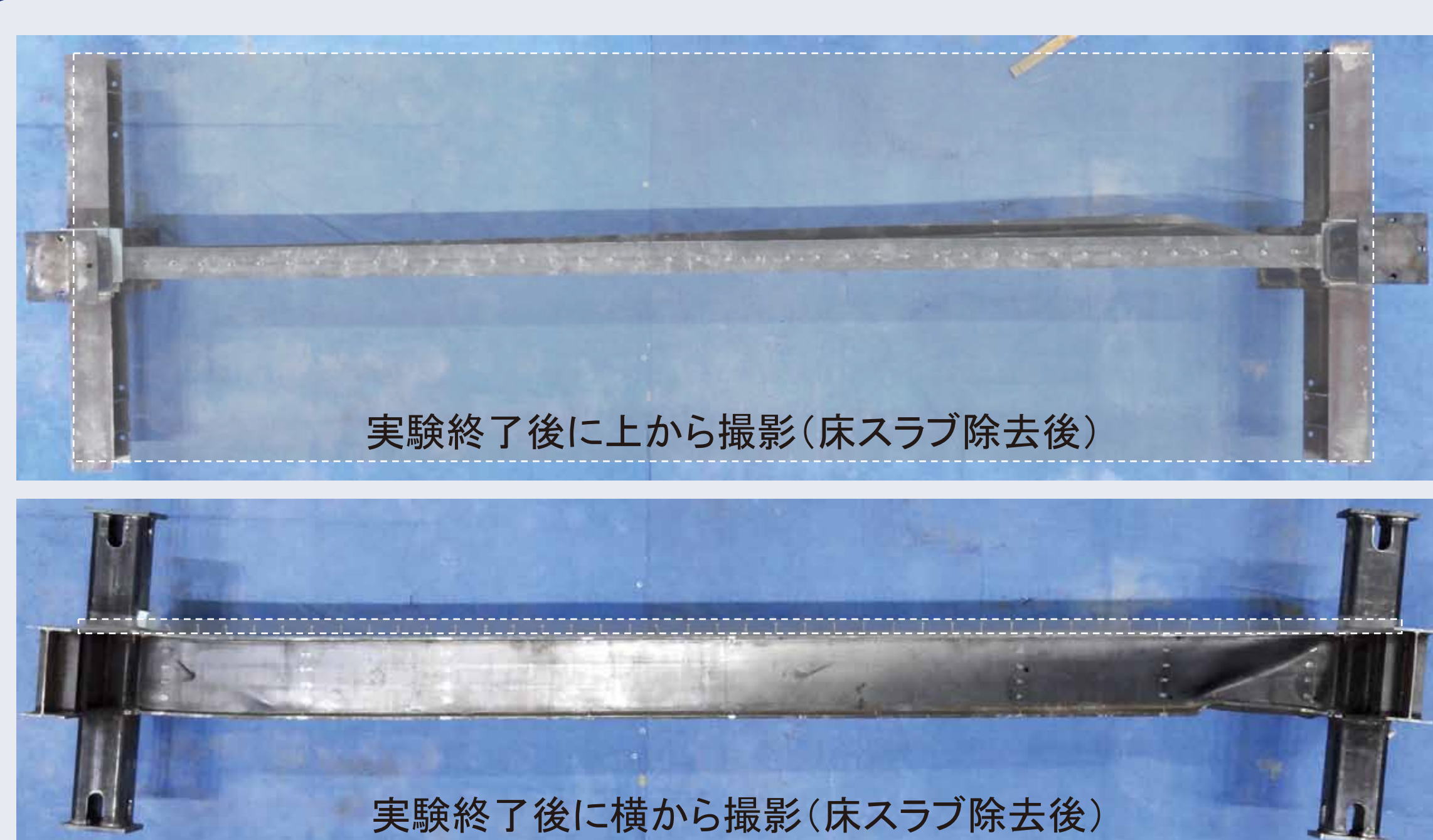
実験結果（スパン6.0m）
