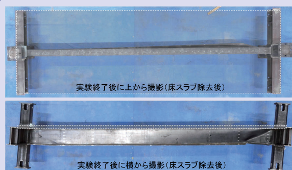
実験結果（スパン6.0m）
