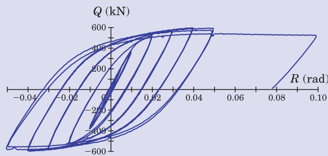
実験結果（スパン6.0m）
